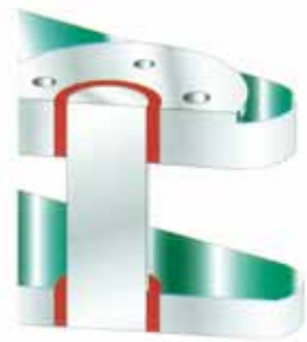
Mise en place de broches/arbres/aiguillot dans d'anciens logements détériorés
